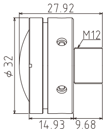
寸法図
